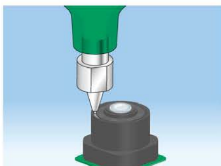
カメラレンズへのUV接着剤塗布
