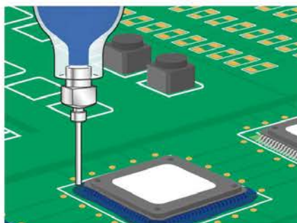
QFPへの防湿剤塗布
