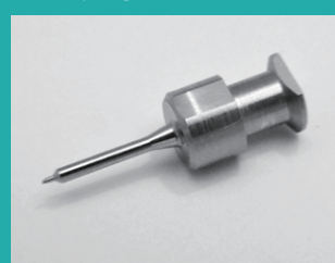
11 1条2段 先細ノズル
