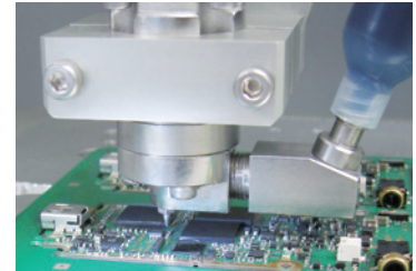
半導体パッケージにアンダーフィル材を塗布
