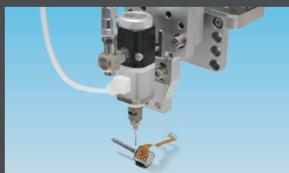
モーター部品にオイルを塗布
