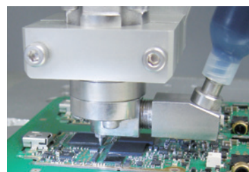
半導体パッケージにアンダーフィル材を塗布
